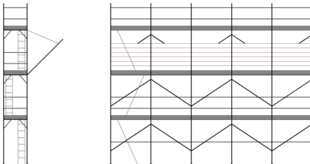
Figura 1 - Prospetto e vista laterale tipo Ponteggio da montare
