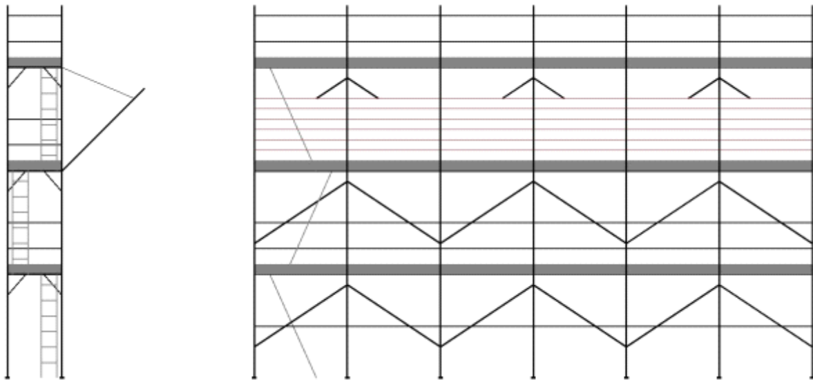
Figura 1 - Prospetto e vista laterale tipo Ponteggio da montare
