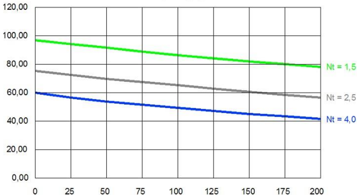
Figura B - Grafico Autoprotezione (Guida CEI 64-17/2010)
